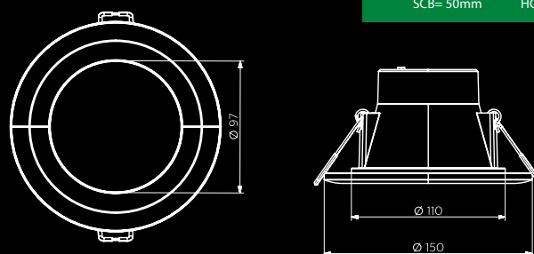
KING D120 Dimensions
