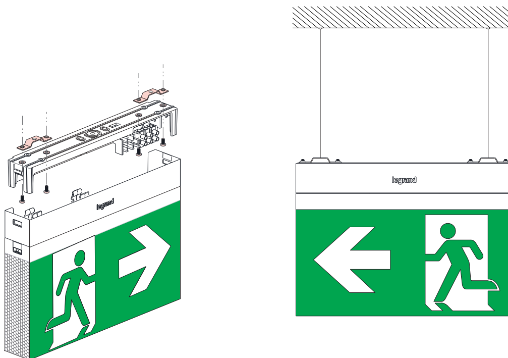
Wire suspension kit (Cat.No: 686216)
