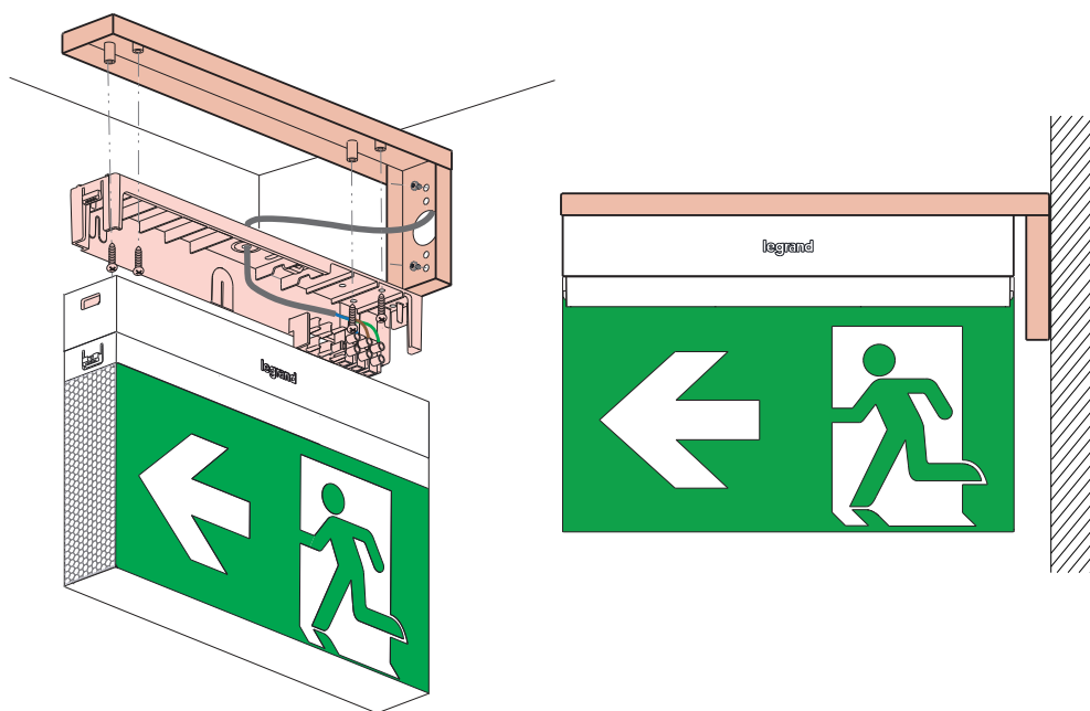
Wall L- bracket (Cat.No: 659459)
