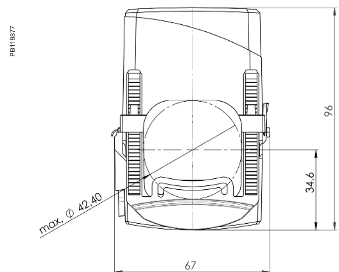
HJ Dimensions
