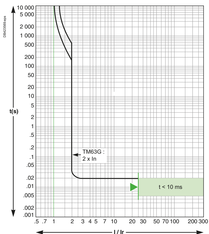
TM63G
