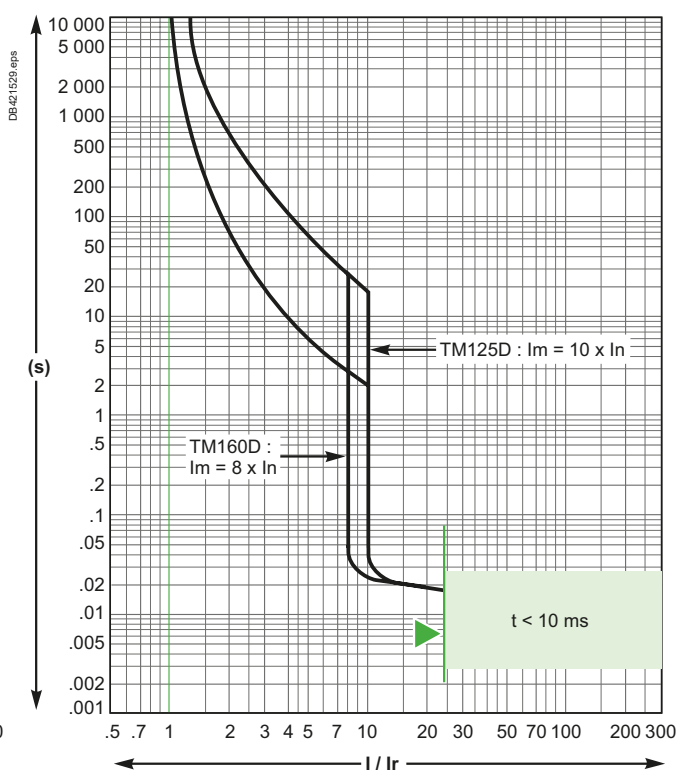
TM125D / TM160D
