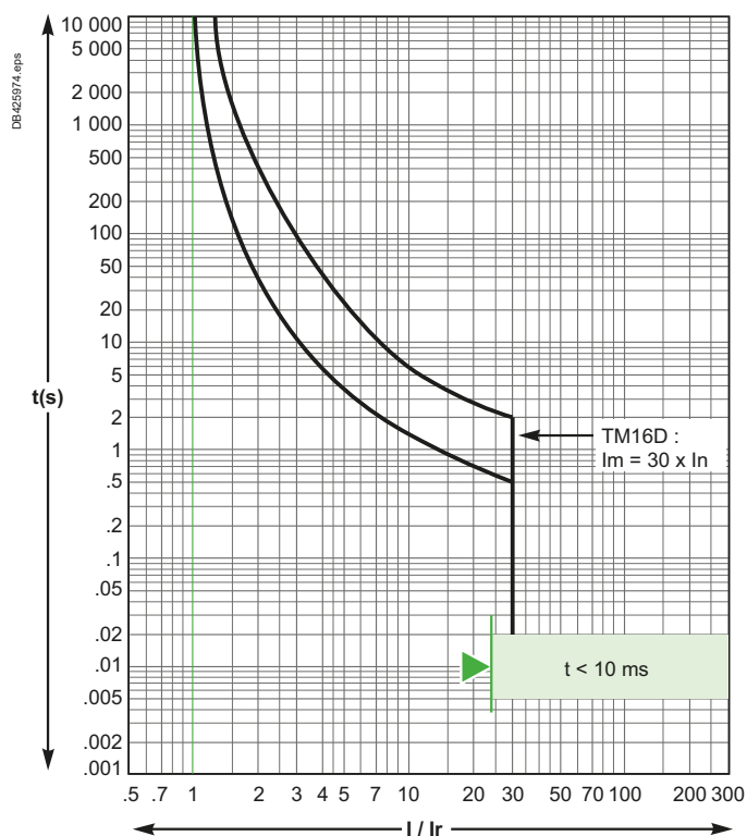
TM16D
