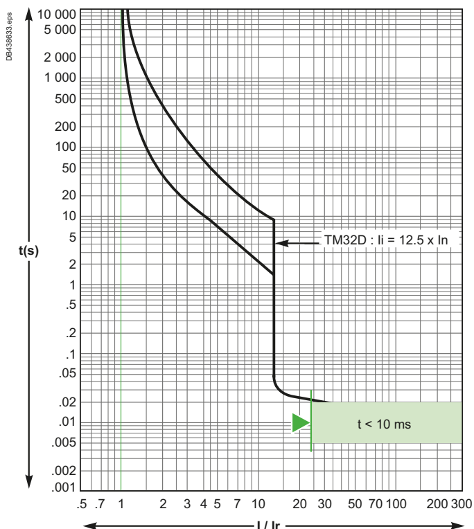
TM30D/TM32D
