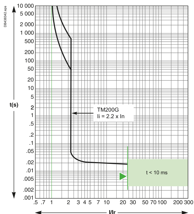
TM200G
